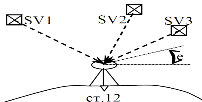
Рис. 1.1. Принцип определения местоположения ГНСС: SV1, SV2 и SV3 – спутники, участвующие в измерениях; e – маска возвышения 10^\circ ; ст. 12 – определяемая точка
