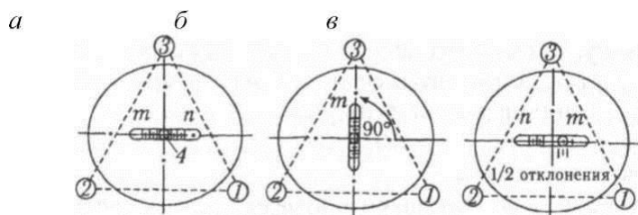
Рис. 2. Поверки цилиндрического уровня: а — установка по двум винтам;
