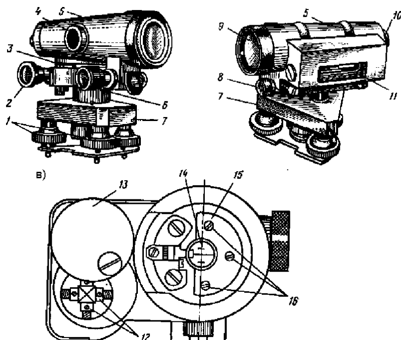
Рис.10 Точный нивелир Н-3:
